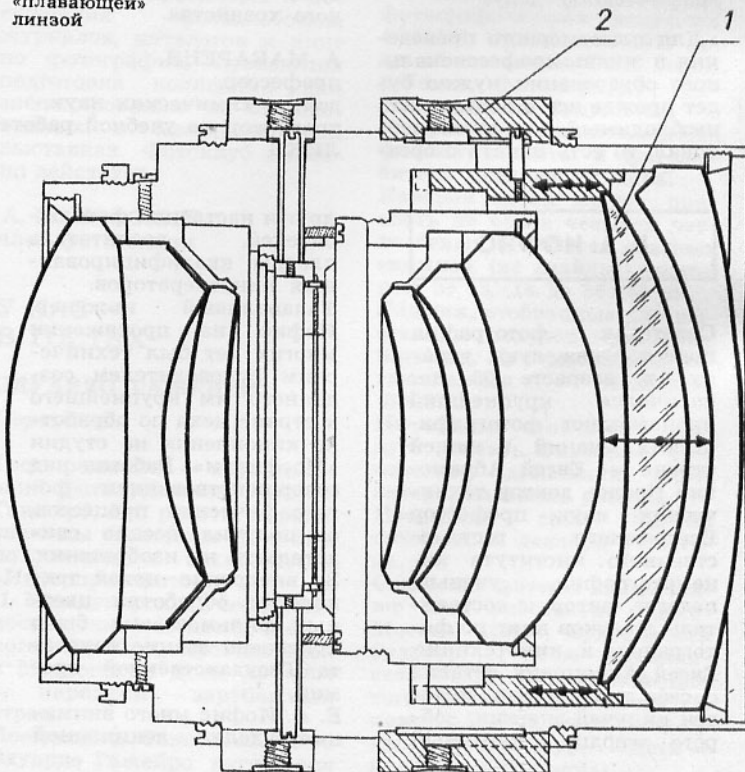
Рис. 1. Схема объектива с «плавающим» оптическим элементом: 1 — «плавающая» линза; 2 — кольцо управления «плавающей» линзой
