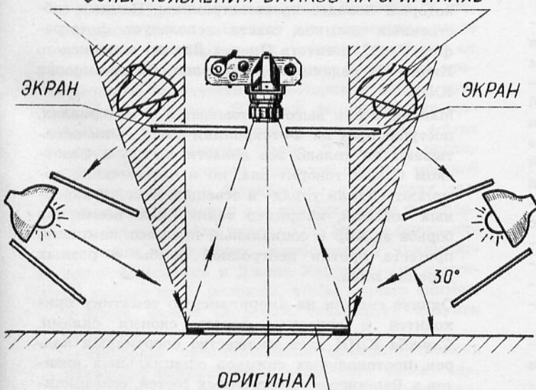
Схема освещения при репродукционной съемке
